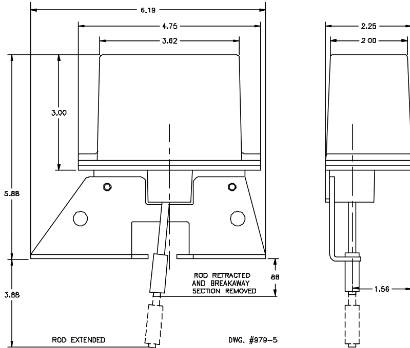
FIG. 3 DIMENSIONS
